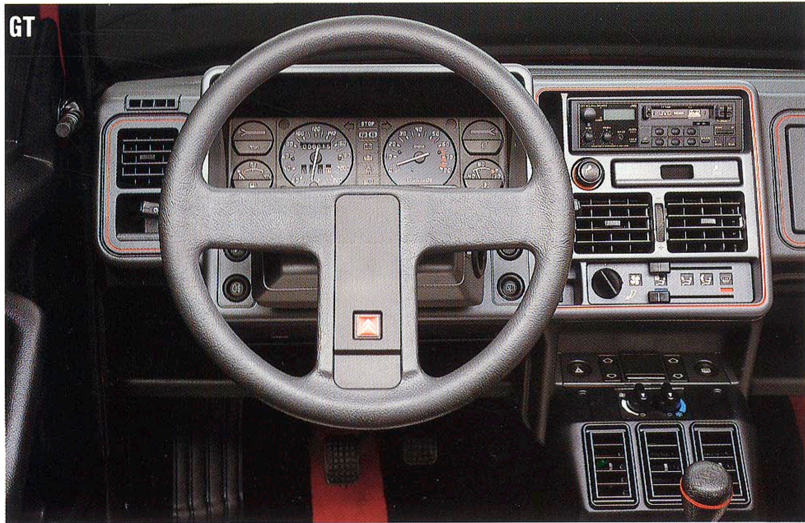
GT 機能性を徹底的に追求したGTのメーターパネル。タコメーターを装備するとともに、右にはエンジン油圧計と水温計、センターには多機能のウォーニング・システムを設置。エンジンの油圧、油量、バッテリー充電、ブレーキパッドの磨耗、サイドブレーキ、ガソリンレベルの低下を、ドライバーに伝達します。またハンドルは、スポーティな3本スポークタイプを採用しています。
