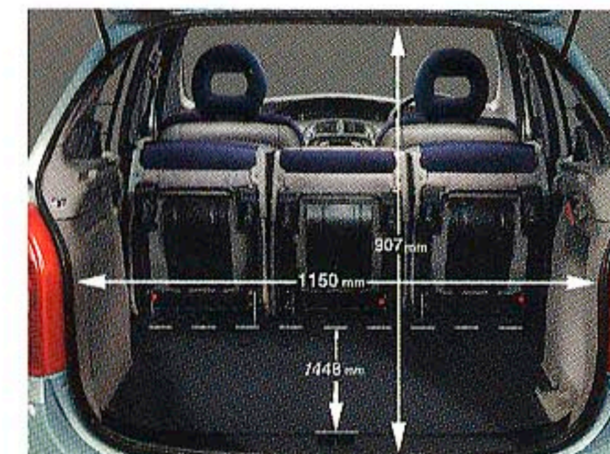
ラゲッジルーム リアシートを倒して折りたためば、1,969ℓもの広大なスペースが出現。荷物がたっぷり積み込めます。
