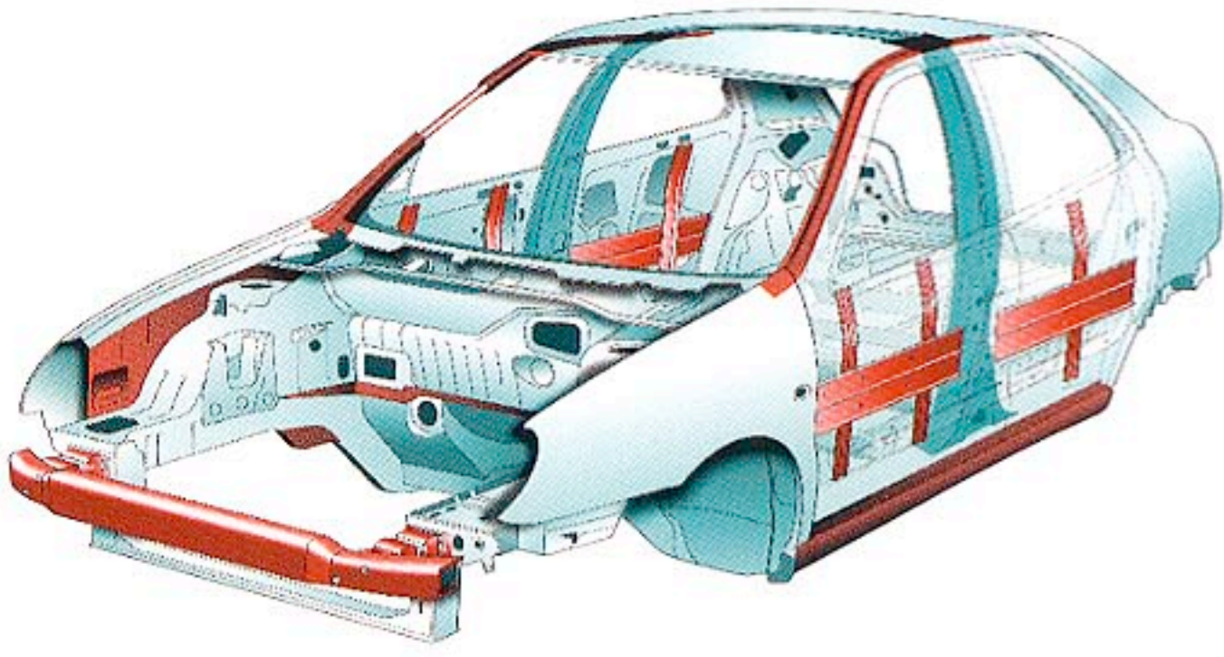
ドア内のサイドインパクトバーの採用をはじめ、 側面および前方からの衝撃に対しボディ剛性を強化
